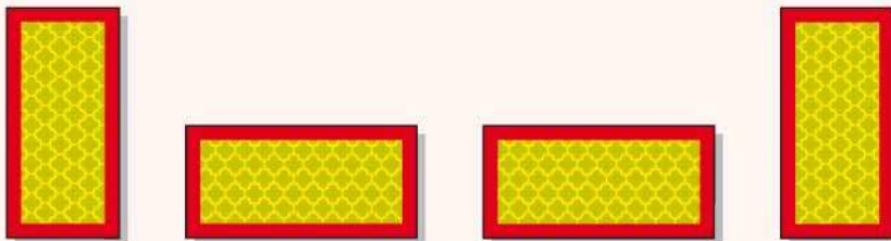
Afmetingen / Dimensions : 283x135mm Aluminium 1mm-Vlak / Plat 2444.04 Geprofileerd / Profile 2425.00
